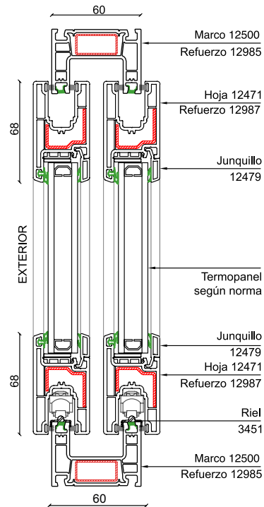
Detalle 1
